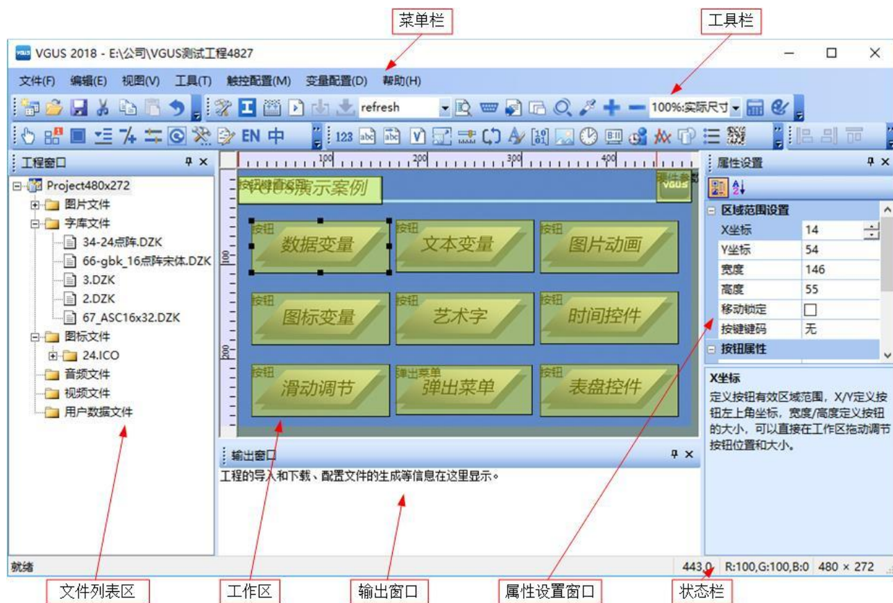
图 7-1-1 VGUS 开发工具软件界面
